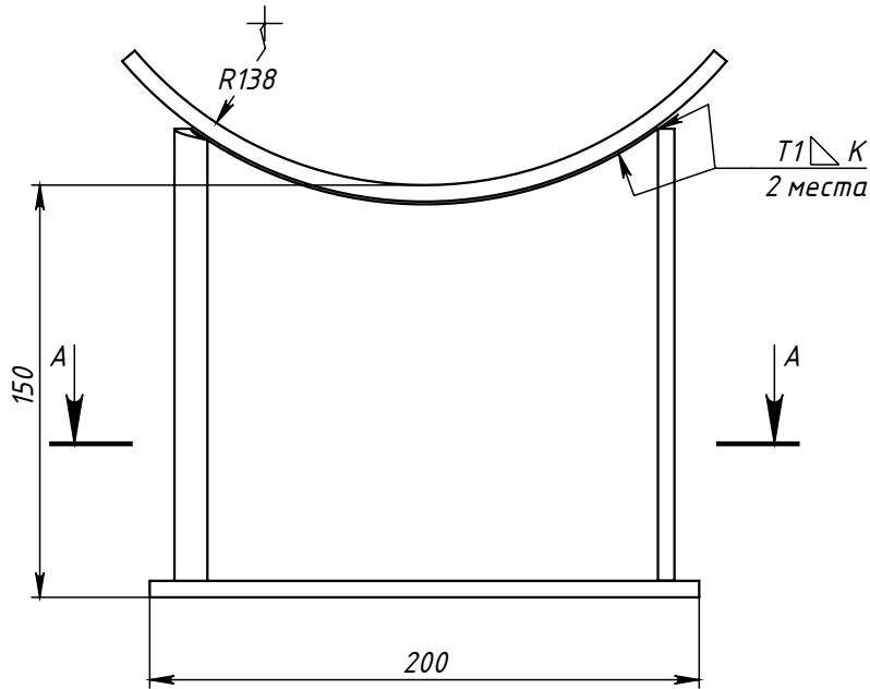
Поз.3 (Ложемент)
