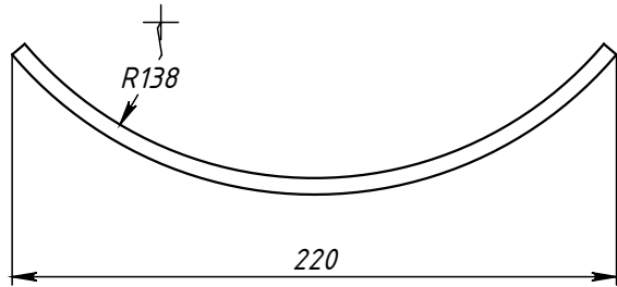
Поз.3 (Ложемент)
